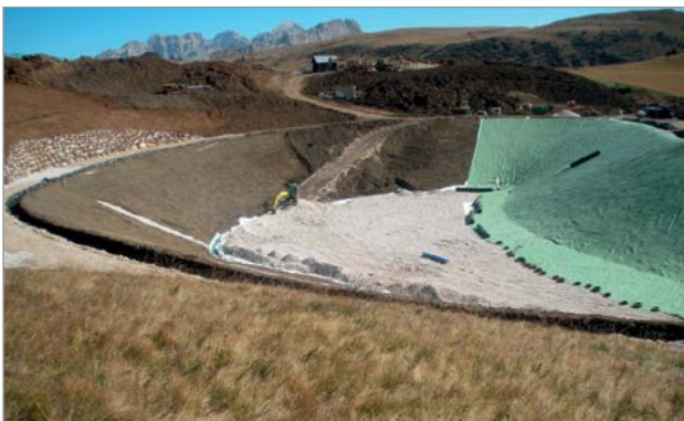
Posa dell'impermeabilizzazione
