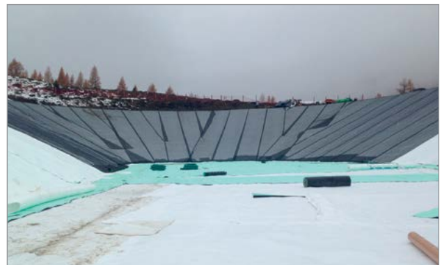
Posa geogriglia tridimensionale Fortrac 3D
