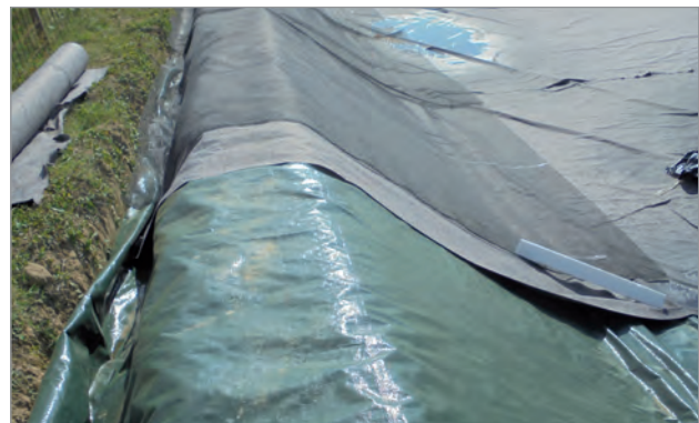
Posa di TNT e Fortrac 3D®-30 sulle sponde
